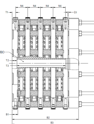
CONJUNTO COM 4 DISCOS 4XX
