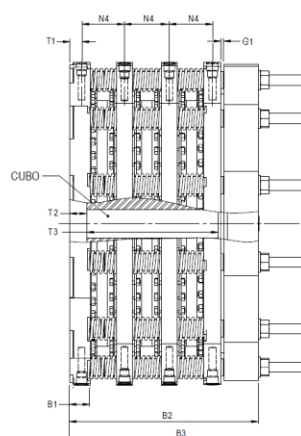
CONJUNTO COM 3 DISCOS 3XX
