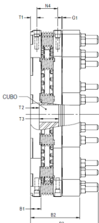
CONJUNTO COM 1 DISCO 1XX
