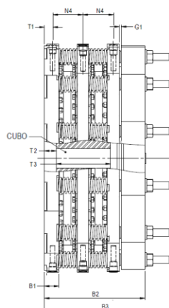
CONJUNTO COM 2 DISCOS 2XX
